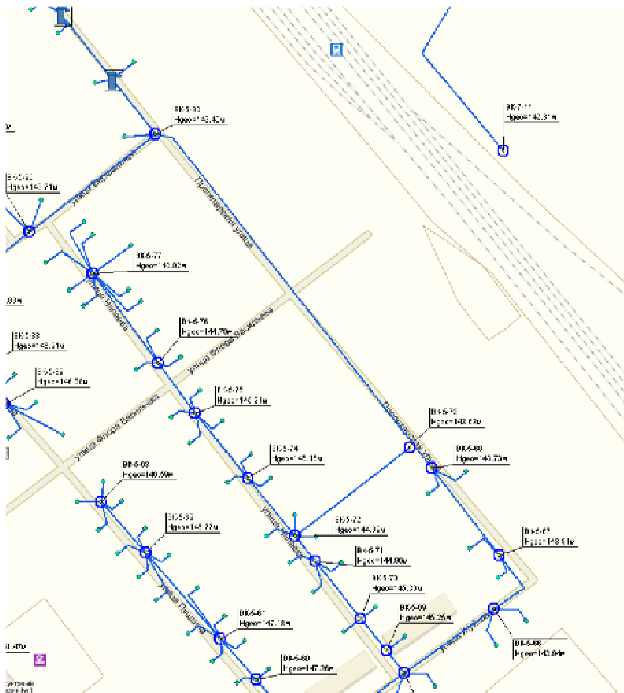
Рисунок 17 – Участки предлагаемые для закольцовки существующих сетей водоснабжения (BK-6-768; BK-5-93)
