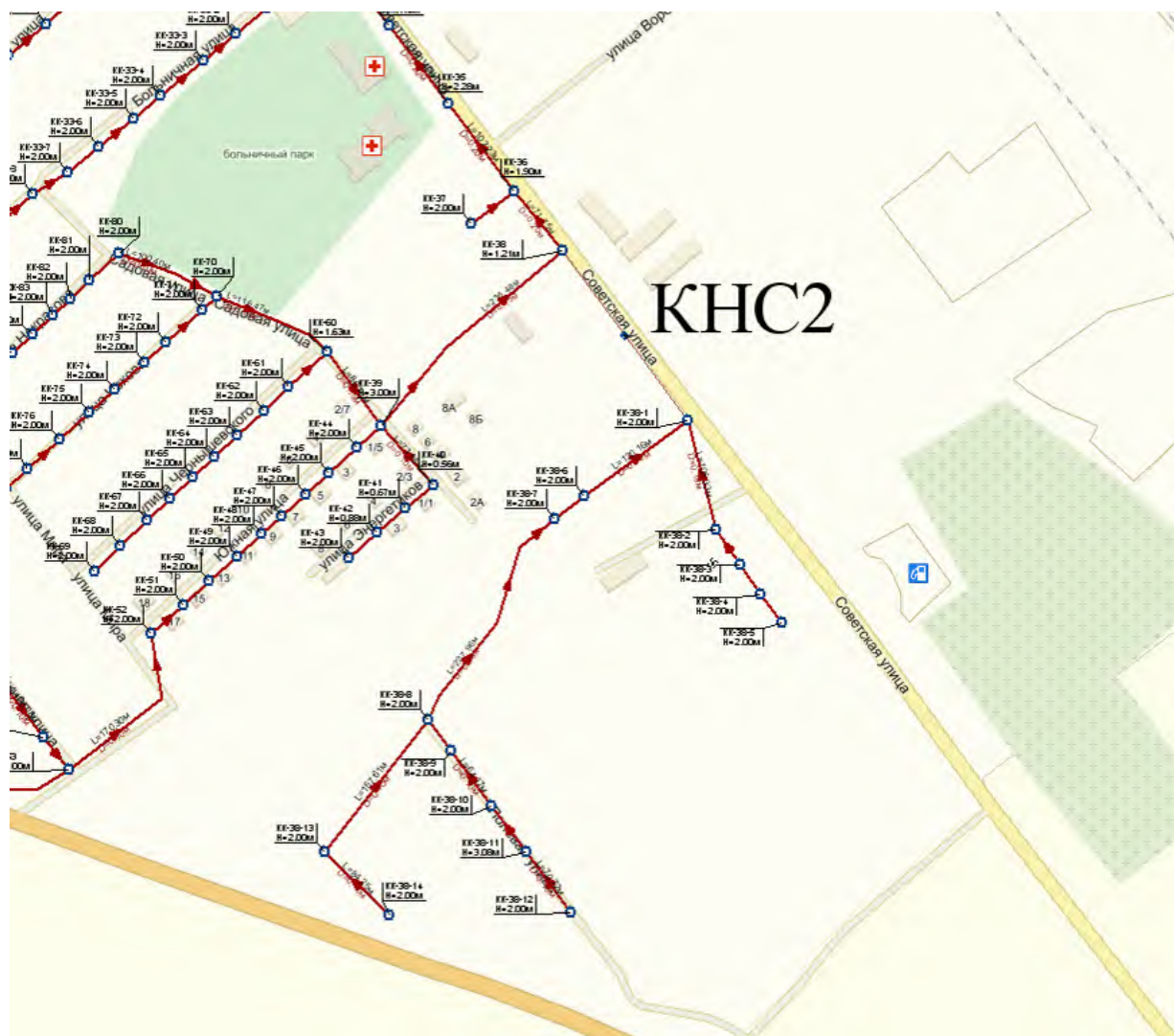
Рисунок 21 - Предлагаемая сеть самотечной канализации в КНС-2 в п. Яр.
