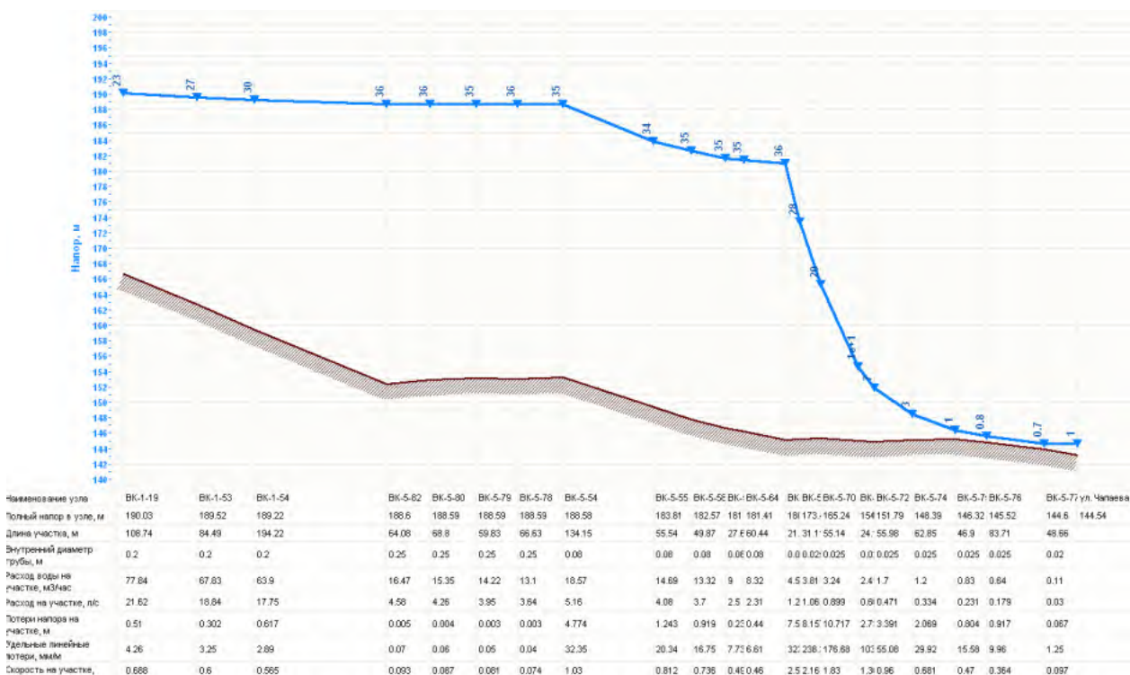
Рисунок 12 – Распределение давления в сети от ВК-1-19 до самого неблагоприятного потребителя по ул. Чапаева
