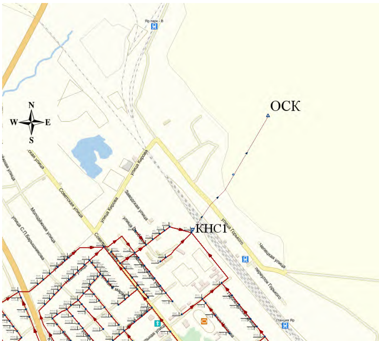
Рисунок 20 - Предлагаемая сеть напорной канализации от КНС-1 до ОСК в п. Яр
