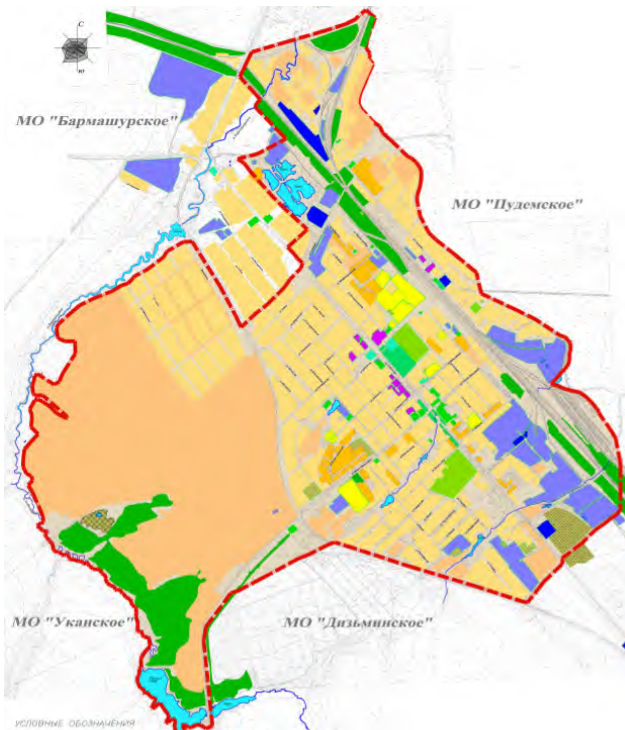
Рисунок 1 – Схема функционального зонирования МО «Ярское»
