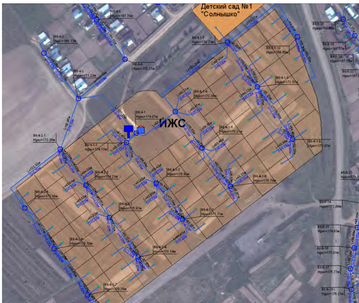
Рисунок 18 – Маршруты прохождения предлагаемых к строительству участков водопроводных сетей на территории перспективной застройки
