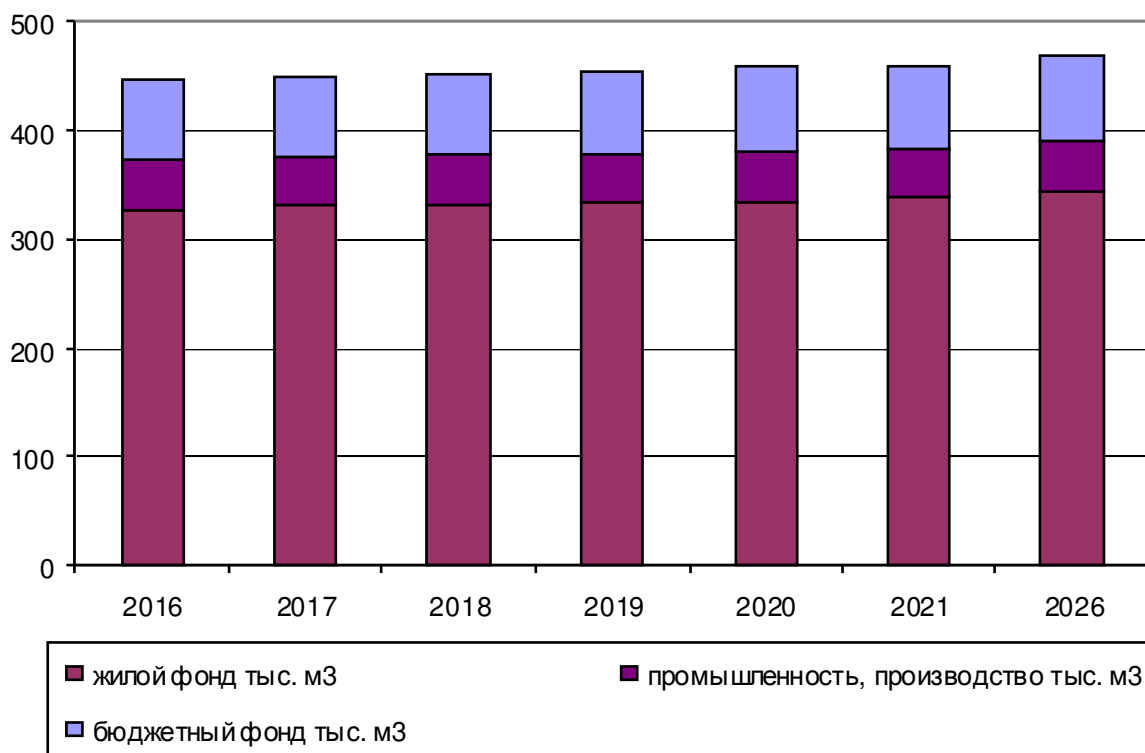
Рисунок 8 – Диаграмма перспективного баланса подачи и реализации воды по структурным составляющим
