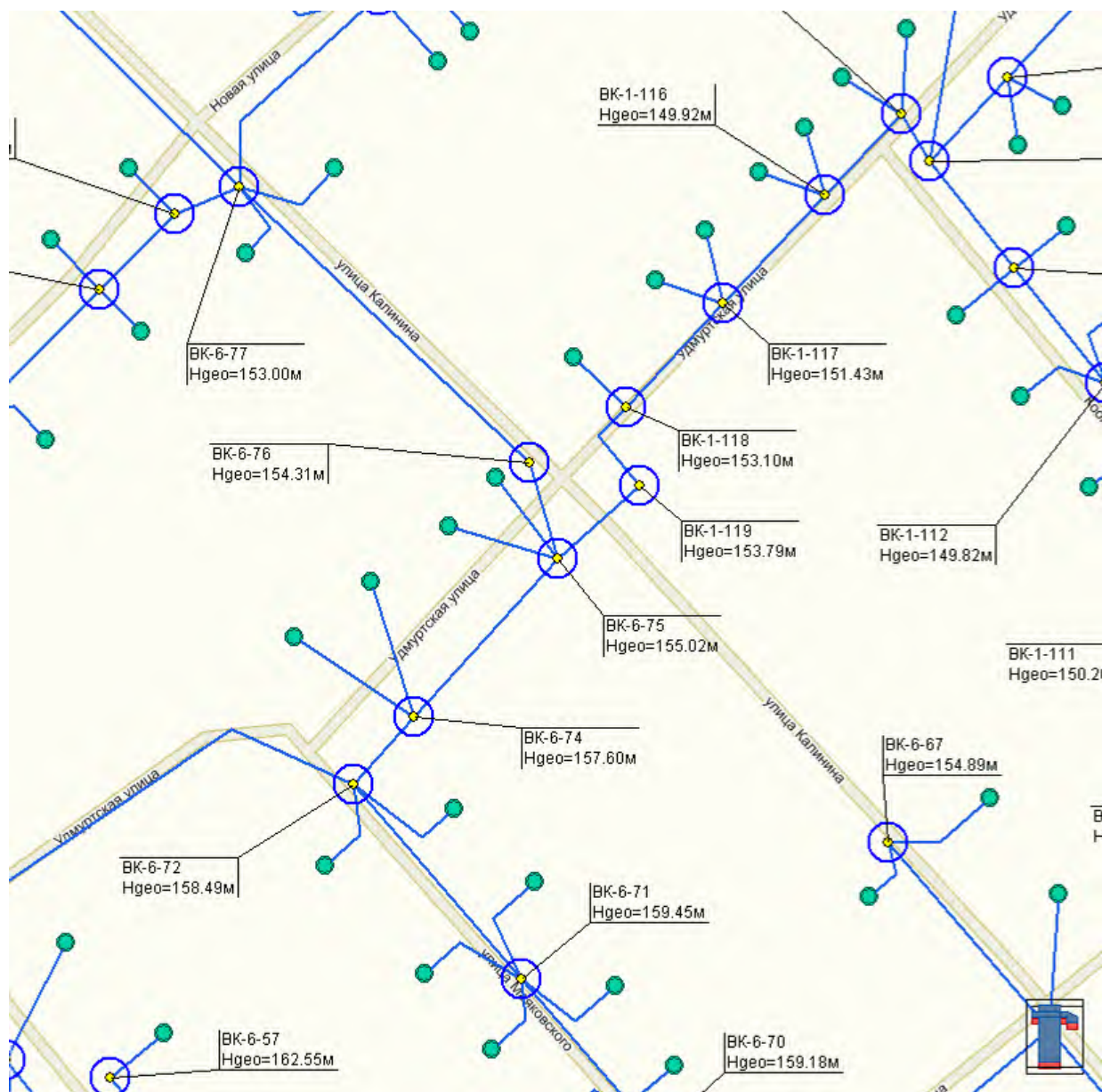
Рисунок 16 – Участки предлагаемые для закольцовки существующих сетей водоснабжения (БК-6-75; БК-1-119)
