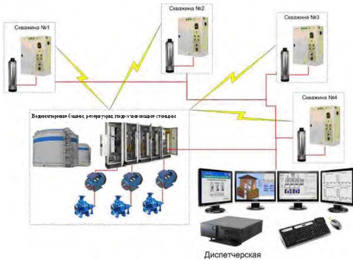
Рисунок 14 – Схема автоматизации, диспетчеризации и управления
