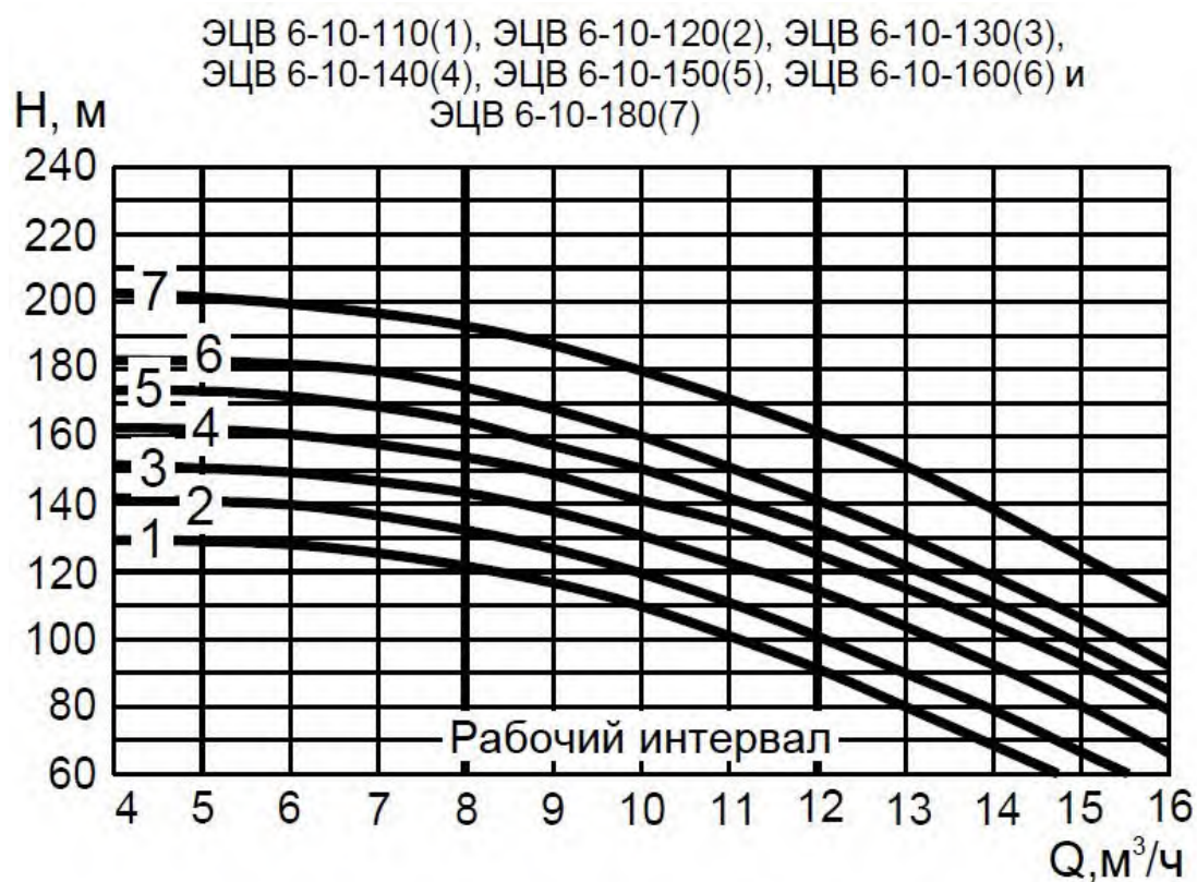
Рисунок 4 – Напорные характеристики насосных агрегатов марки ЭЦВ
