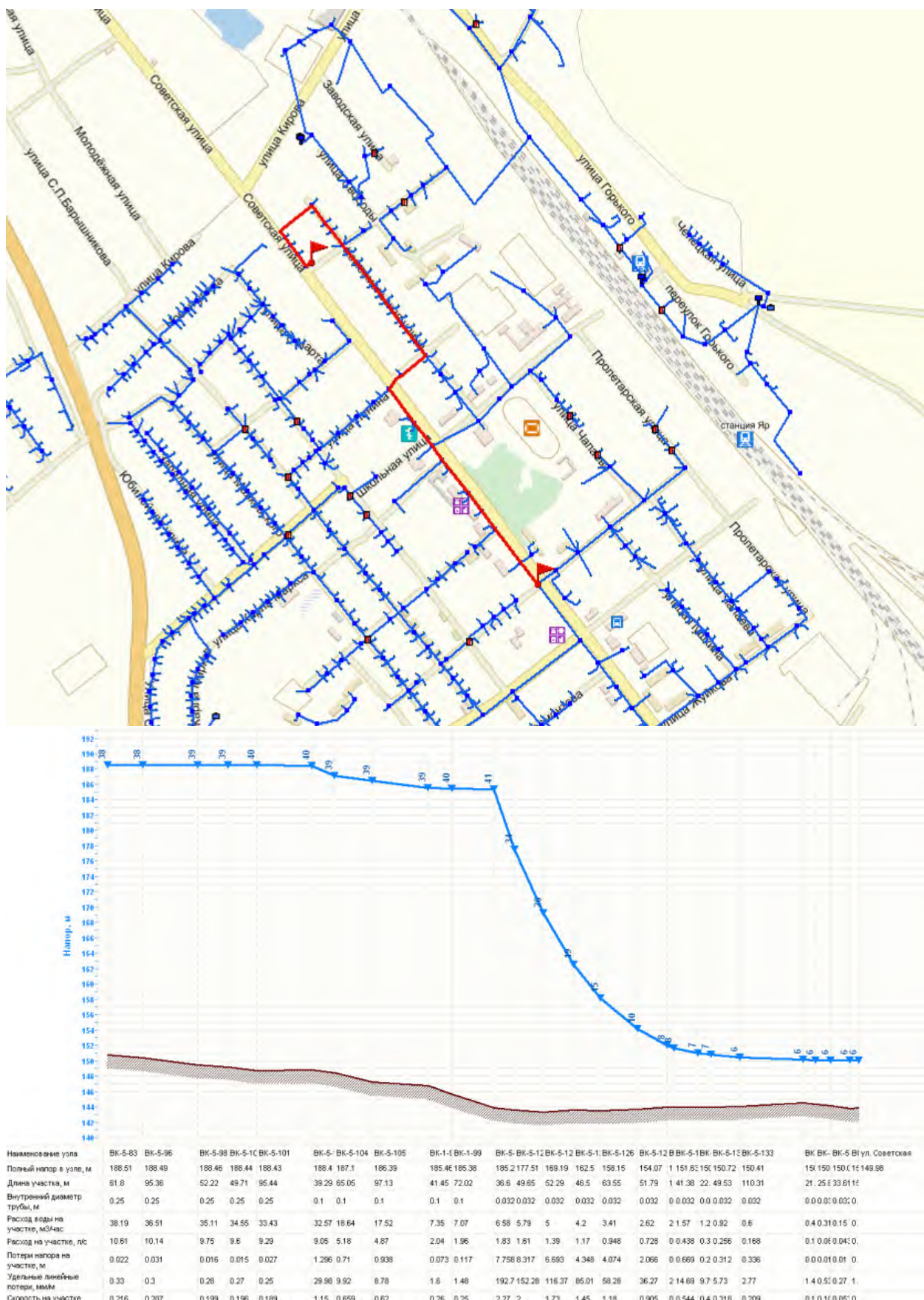
Рисунок 13 – Распределение давления в сети от ВК-5-83 до самого неблагоприятного потребителя по ул. Советская
