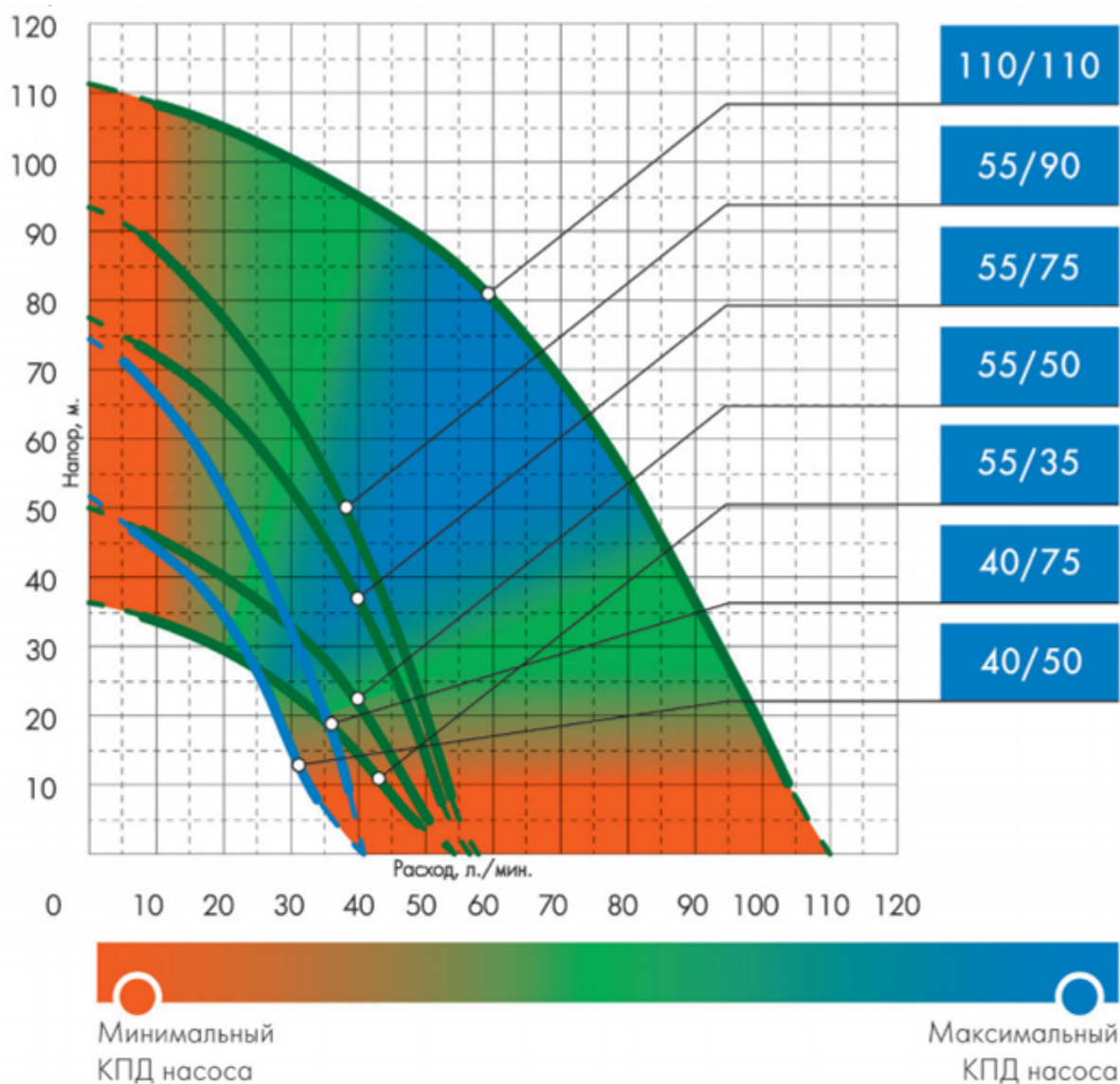
Рисунок 4 – Напорные характеристики насосных агрегатов марки Водомет Проф
