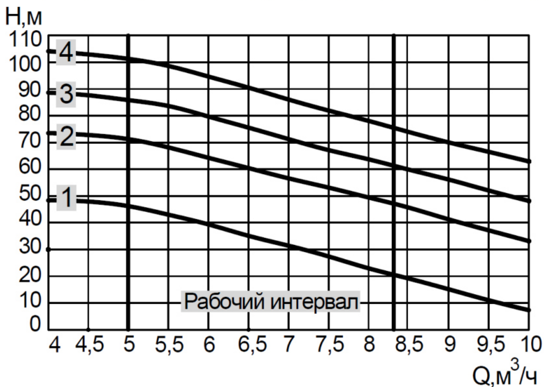
ЭЦВ 6-6,5-35(1), ЭЦВ 6-6,5-60(2), ЭЦВ 6-6,5-75(3) и ЭЦВ 6-6,5-90(4)
